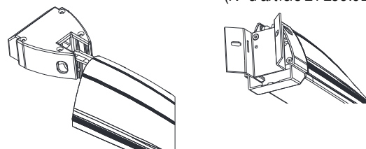
Fixation sur poteau ou sur coin (Aero, Aero-868/ Aero-868 Plus) Accessoire optionnel (N° d'article 24 269.020 1)
